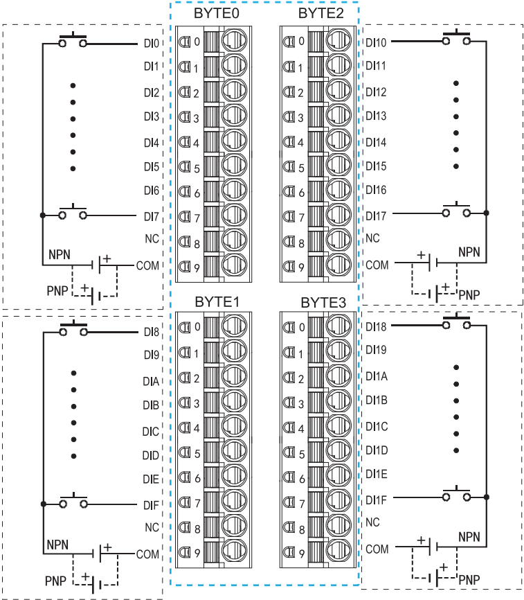
点位分布及外部接线图 输入端子
