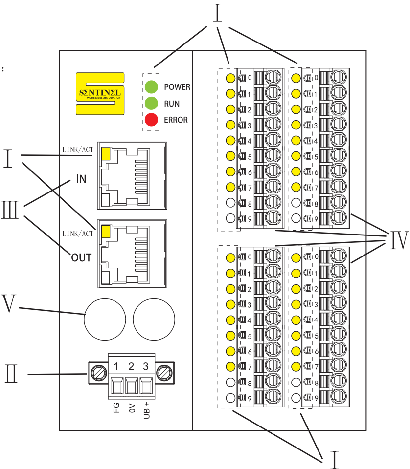
点位分布及外部接线图 输入端子
